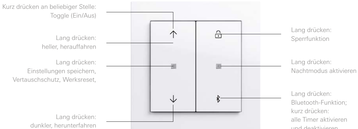
Gira Jalousie- und Schaltuhr BT
