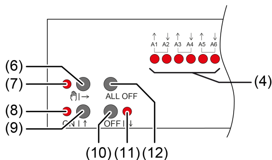
Bild 2: Bedienelemente
