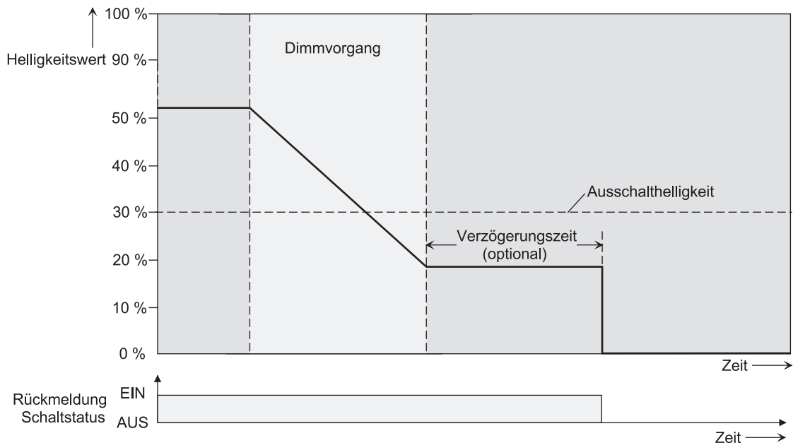
Bild 38: Dimm- und Schaltverhalten der automatischen Ausschaltfunktion
