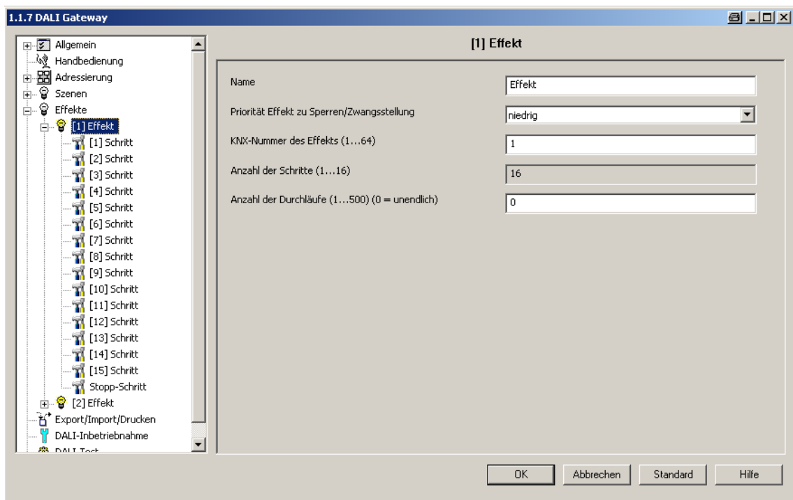
Bild 52: Konfigurationsseite eines Effekts als Beispiel mit 15 angelegten Effekt-Schritten und Stopp-Schritt
