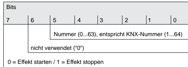
Bild 55: Struktur des Objektwerts für die Effekt-Nebenstelle
