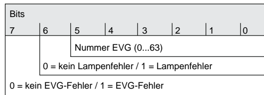
Bild 30: Telegrammaufbau 1 Byte Fehlerstatus
