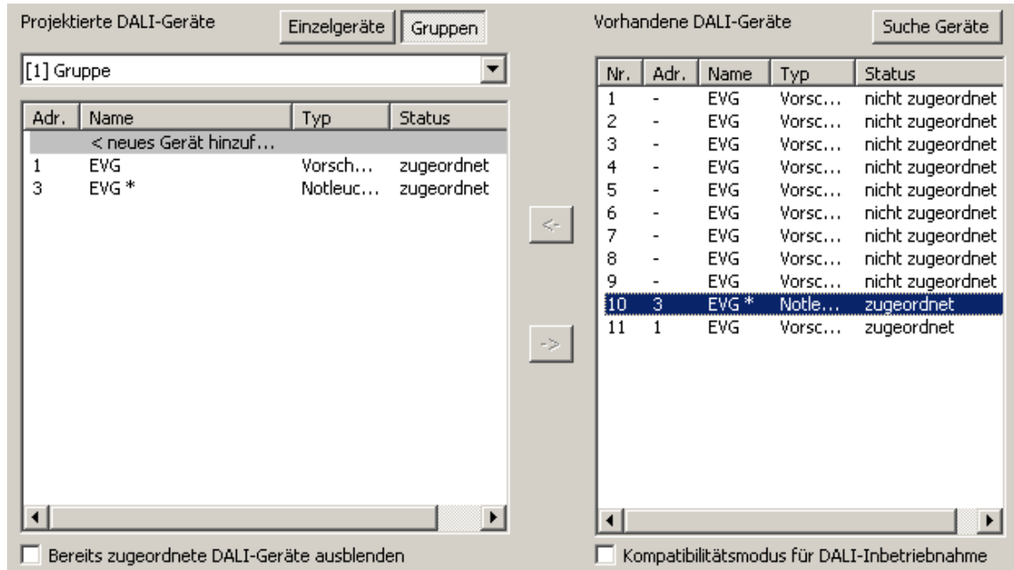
Bild 66: Betriebsgerät einer Gruppe zugeordnet Hier: EVG mit Adresse 3 ist mehreren Gruppen zugeordnet.
