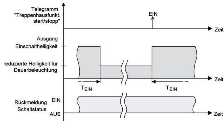
Bild 46: Die Dauerbeleuchtung der Treppenhausfunktion ohne Soft-Funktionen
