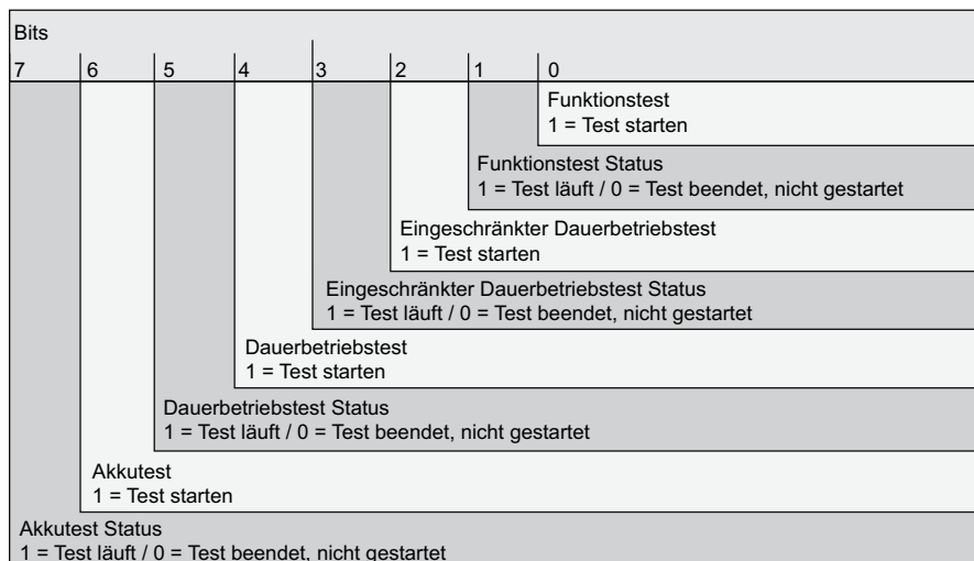
Bild 57: Struktur des 1 Byte Objekts "Notbetrieb Test Start / Status"
