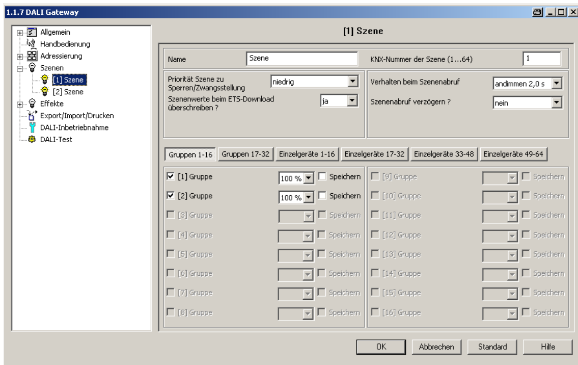
Bild 50: Konfigurationsseite einer Szene als Beispiel mit zwei angelegten Szenen und zwei DALI-Gruppen
