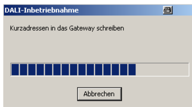
Bild 69: Abgleich der Inbetriebnahmeparameter zwischen Plug-In und DALI-Gateway. Hier: Einprogrammieren der Kurzadressen
