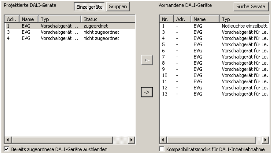
Bild 67: Betriebsgerät einem projektierten Einzelgerät zugeordnet
