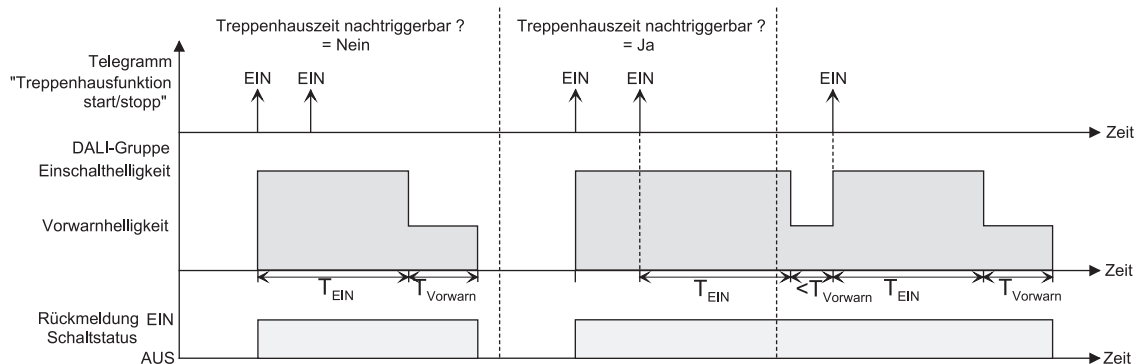
Bild 40: Einschaltverhalten der Treppenhausfunktion ohne Soft-Funktionen
