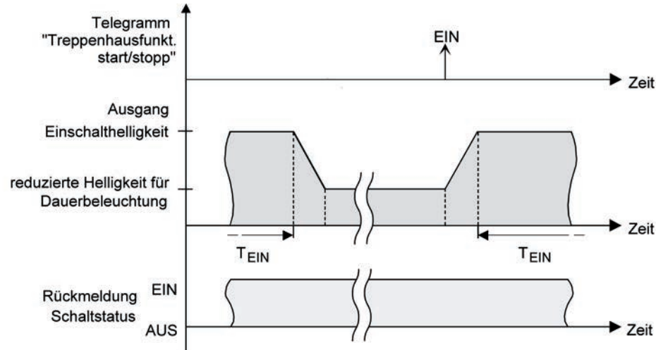
Bild 47: Die Dauerbeleuchtung der Treppenhausfunktion mit Soft-AUS-Funktion
