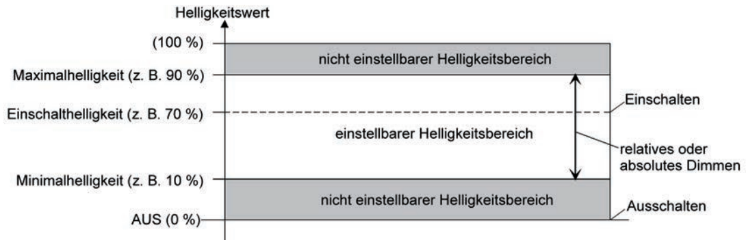
Bild 36: Einstellbarer Helligkeitsbereich beim Dimmen (Beispiel)
