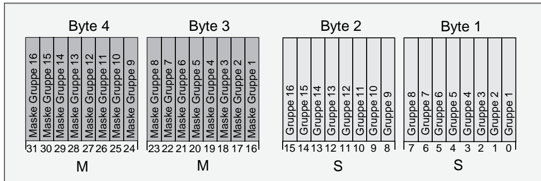
Bild 32: Struktur der Objekte der Sammelrückmeldung am Beispiel des Objekts für die Gruppen 1-16
