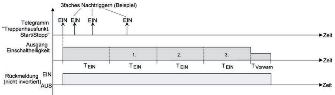
Bild 48: Zeitverlängerung der Treppenhausfunktion
