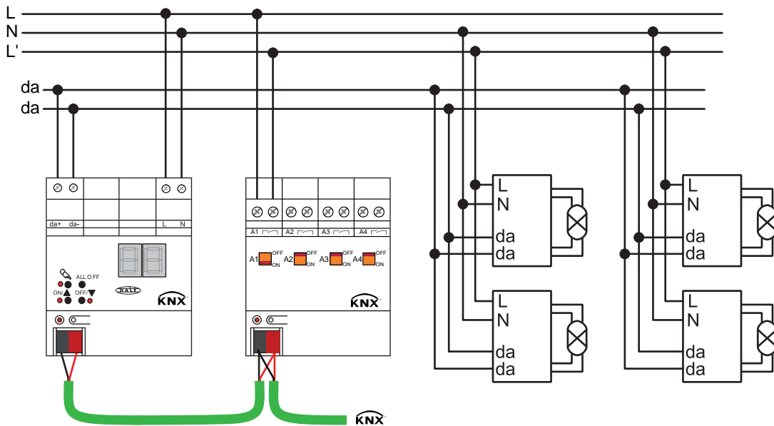
Bild 33: Beispiel eines Anschluss-Schemas zur Standby-Abschaltung durch einen KNX-Schaltfaktor
