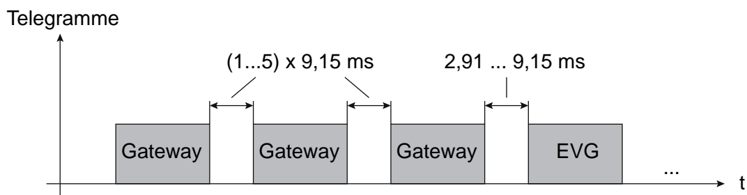
Bild 29: Pausenzeiten zwischen DALI-Telegrammen
