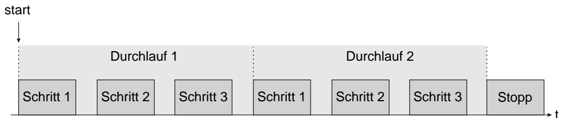
Bild 53: Beispiel eines Effekt-Durchlaufes mit automatischem Stopp (hier: 3 Effekt-Schritte, 2 Durchläufe)
