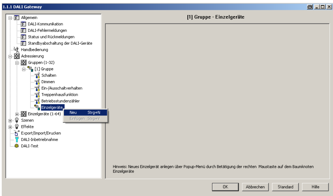
Bild 71: Zuordnen eines EVG zu einer Gruppe - Offline-Inbetriebnahme
