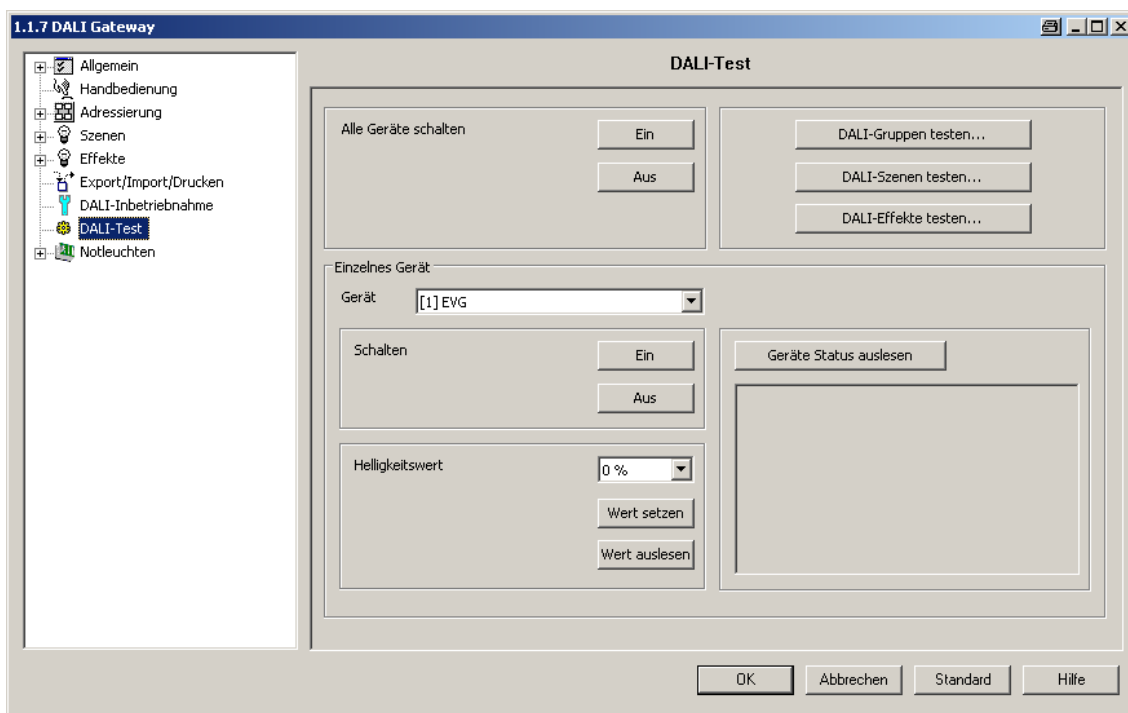
Bild 74: DALI-Testumgebung im ETS3 Plug-In
