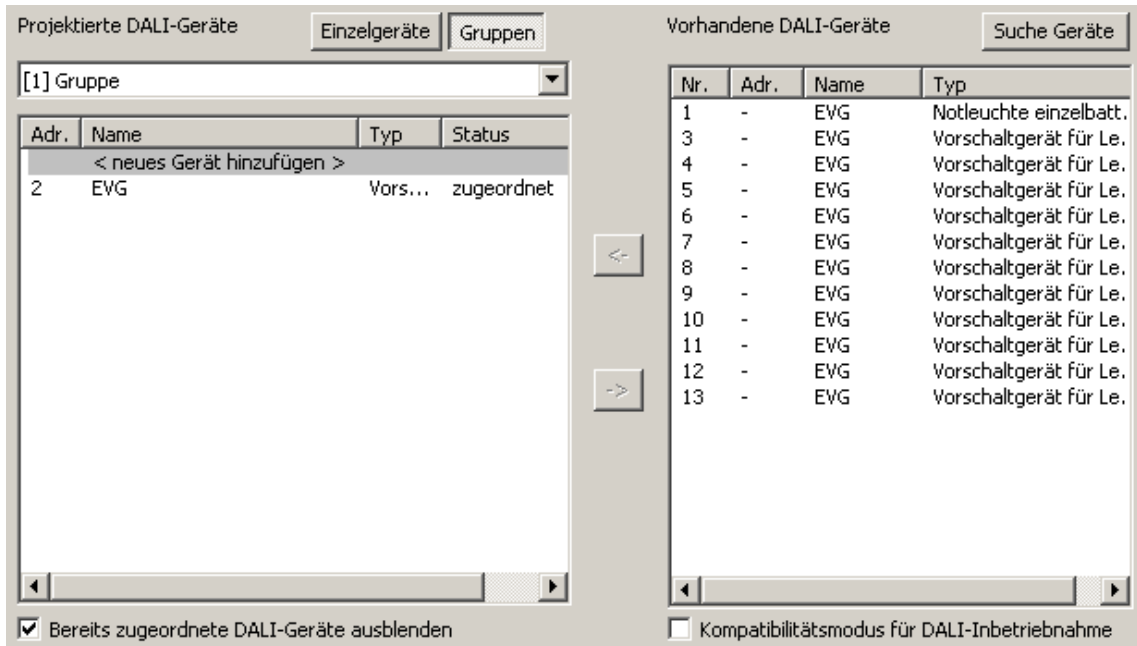
Bild 65: Betriebsgerät einer Gruppe zugeordnet
