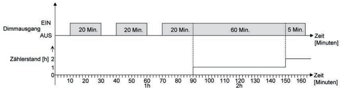
Bild 49: Funktionsweise des Betriebsstundenzählers (am Beispiel eines Vorwärtzählers)
