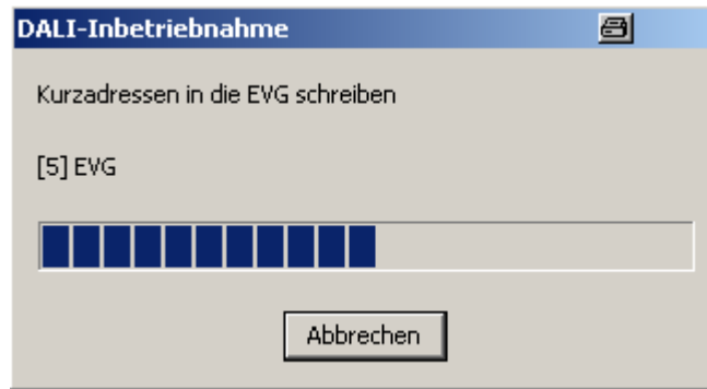
Bild 70: Abgleich der Inbetriebnahmeparameter zwischen Gateway und den DALI-Betriebsgeräten.
