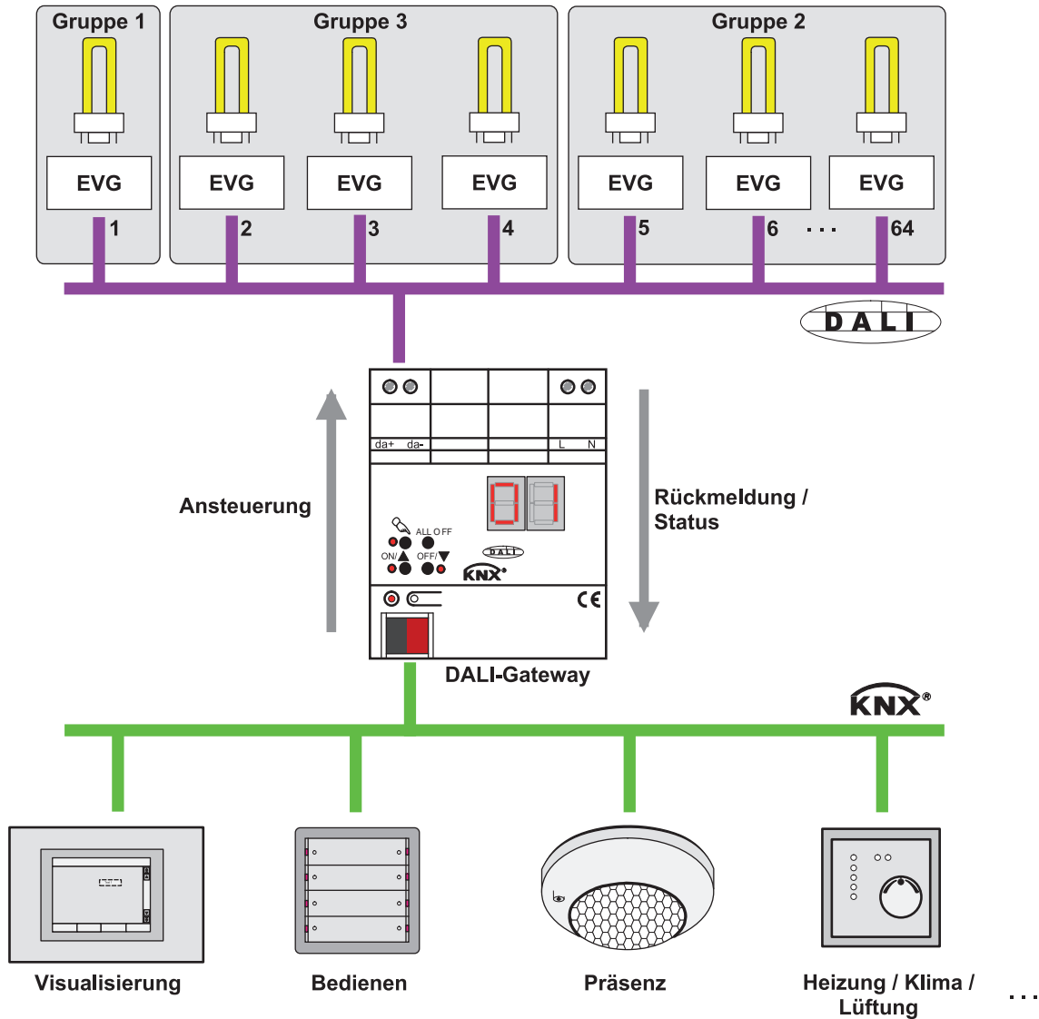
Bild 9: Prinzipübersicht einer KNX-DALI-Systemanbindung (Beispiel)
