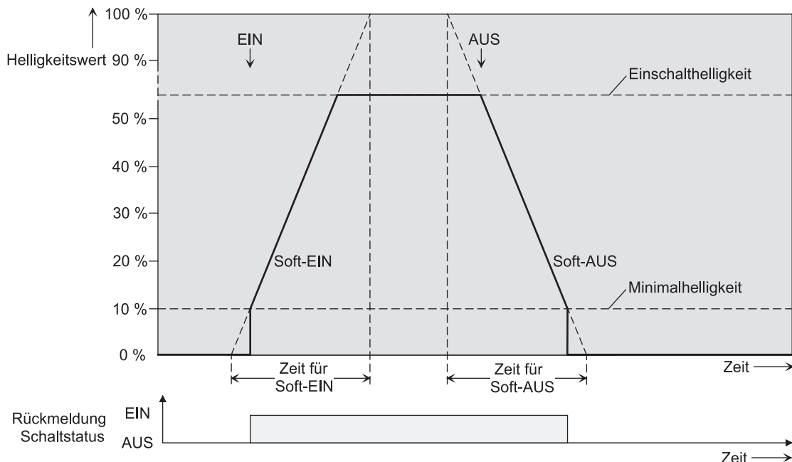
Bild 39: Dimmverhalten der Soft-EIN/AUS-Funktionen als Beispiel mit Minimalhelligkeit > 0%
