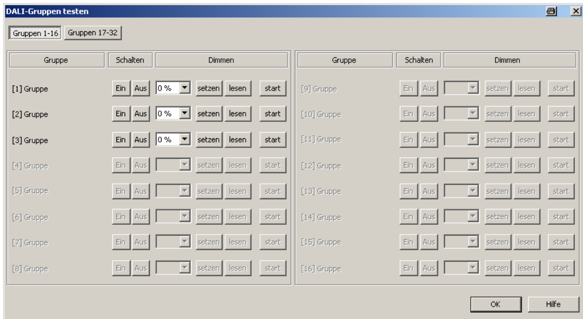
Bild 77: Gruppenorientierte DALI-Testumgebung (als Beispiel mit drei angelegten Gruppen)
