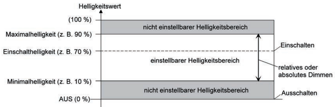
Bild 34: Beispiel eines Helligkeitsbereichs mit Einschalthelligkeit
