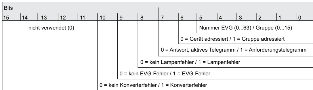
Bild 31: Telegrammaufbau 2 Byte KNX-Fehlerstatus
