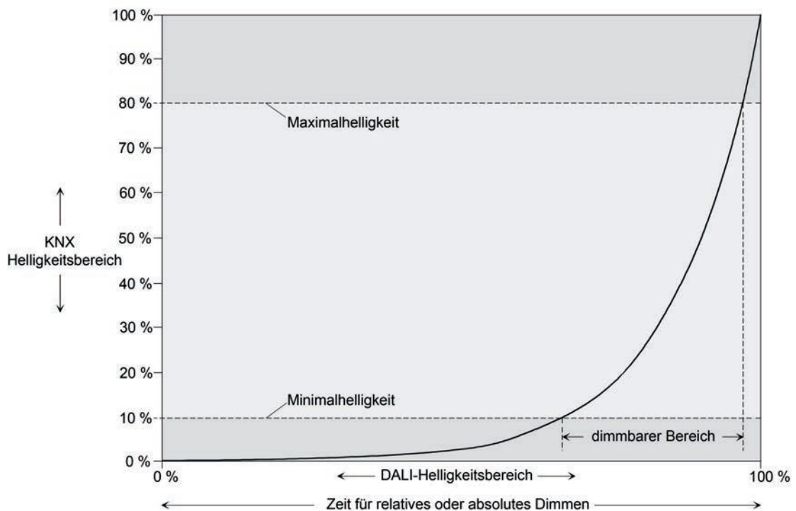
Bild 37: Dimmkennlinie für relatives oder absolutes Dimmen als Beispiel mit Minimal- und Maximalhelligkeit
