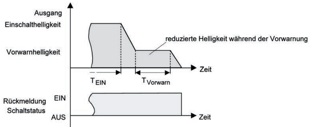
Bild 45: Die Vorwarnfunktion der Treppenhausfunktion mit Soft-AUS-Funktion (als Beispiel mit Minimalhelligkeit = 0 %)
