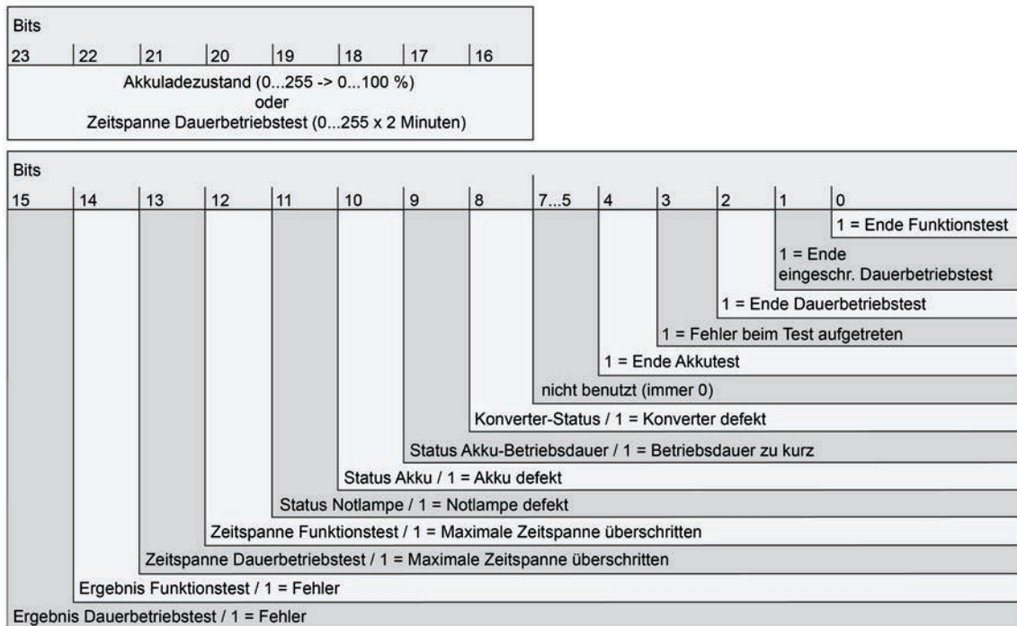
Bild 58: Struktur des 3 Byte Objekts "Rückmeldung Notbetrieb Test"
