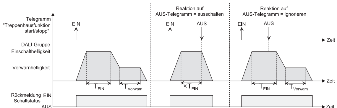
Bild 43: Ausschaltverhalten der Treppenhausfunktion mit Soft-Funktionen (als Beispiel mit Minimalhelligkeit = 0 %)
