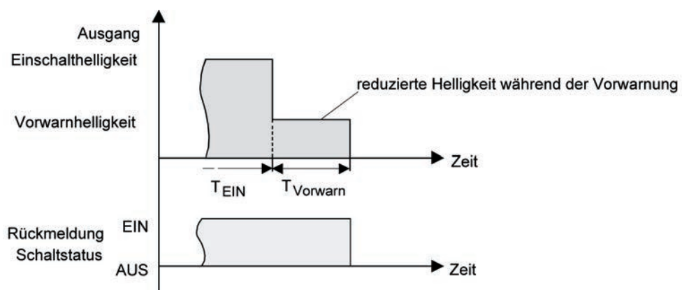
Bild 44: Die Vorwarnfunktion der Treppenhausfunktion ohne Soft-AUS-Funktion
