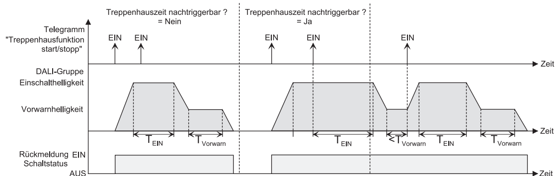
Bild 41: Einschaltverhalten der Treppenhausfunktion mit Soft-Funktionen (als Beispiel mit Minimalhelligkeit = 0 %)
