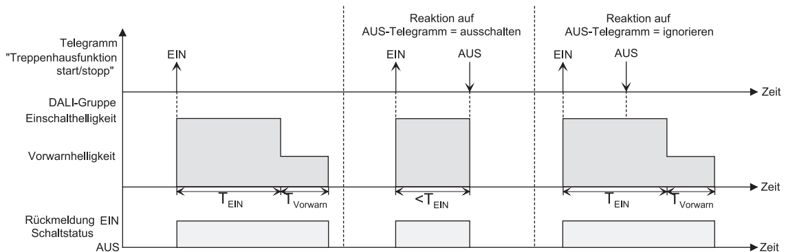
Bild 42: Ausschaltverhalten der Treppenhausfunktion ohne Soft-Funktionen
