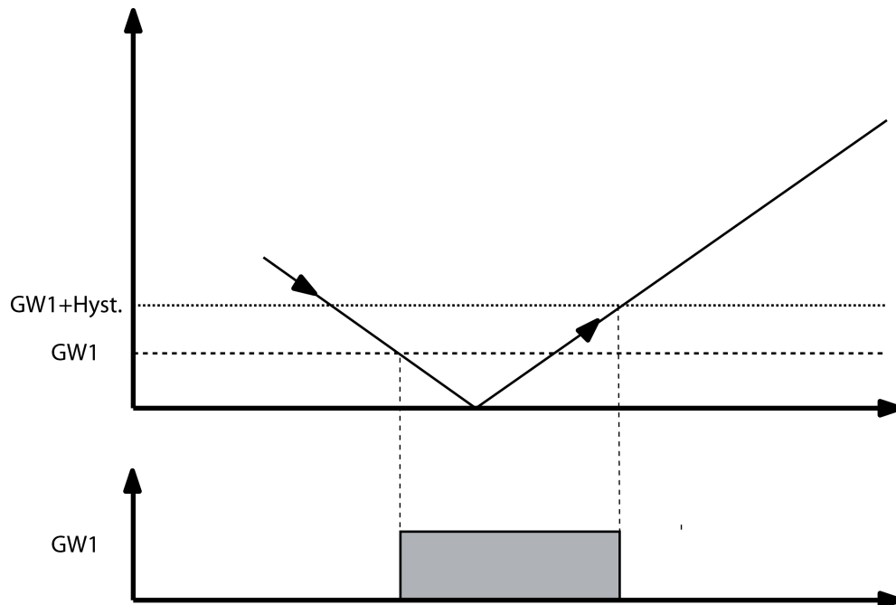
Bild 16: Aktivierung Grenzwert
