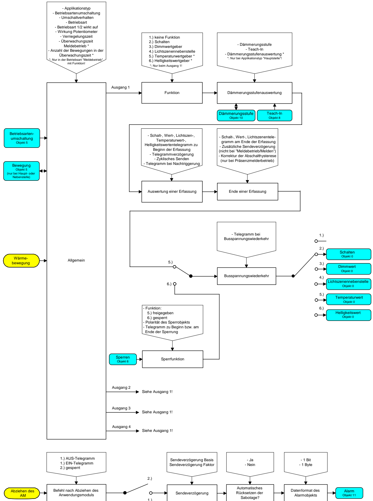
Funktionsschaltbild
